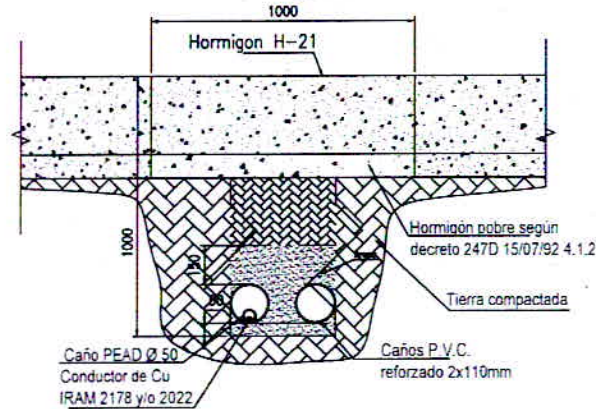
Detalle N°2
