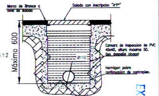
Camara de Paso para cruce de calle
