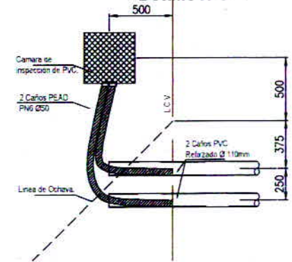
Detalle N°3
