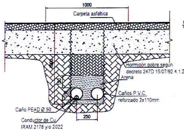
Detalle N°2
