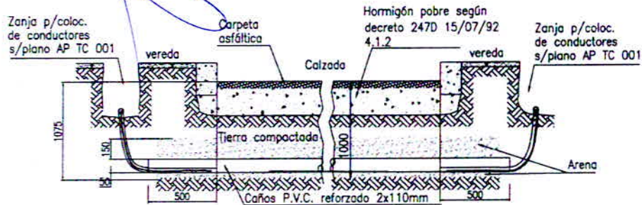
CORTE - CALZADA CON CARPETA ASFALTICA
