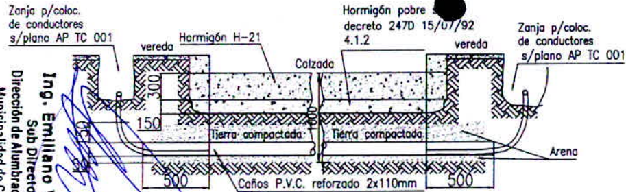
CORTE - CALZADA DE HORMIGON
