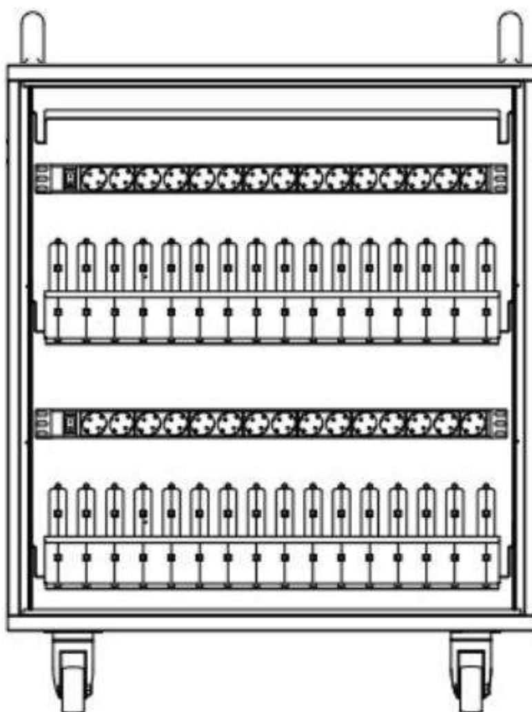
VISTA TRASERA
