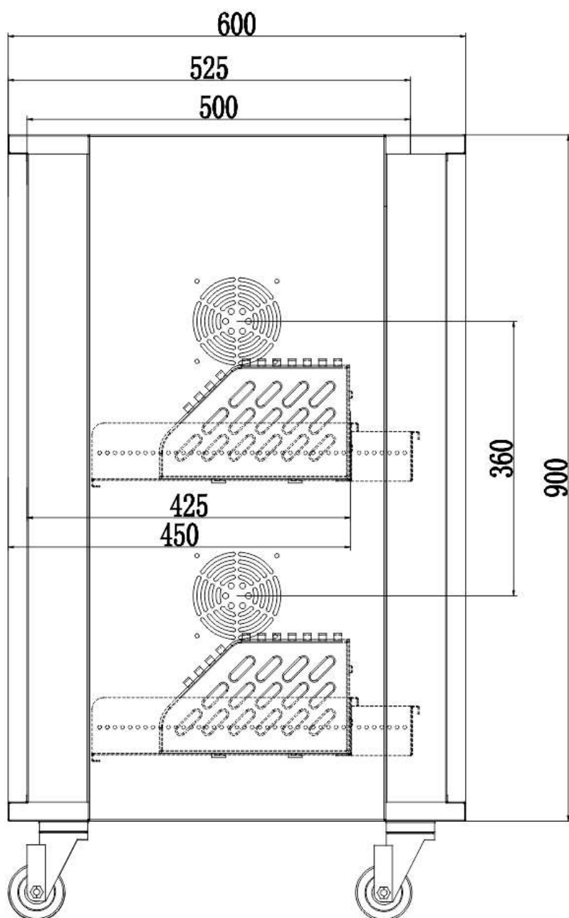
VISTA LATERAL
