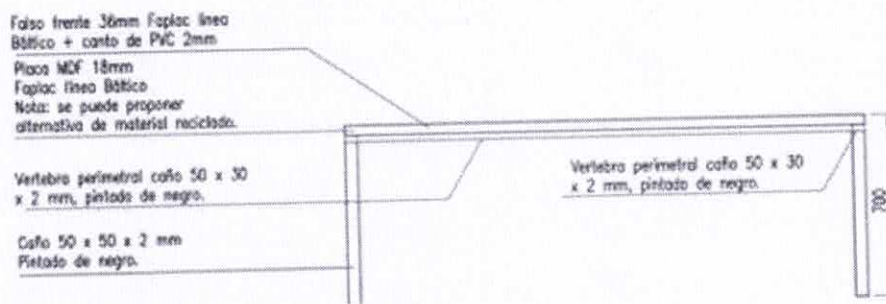
VISTA 1 MOBILIARIO D
