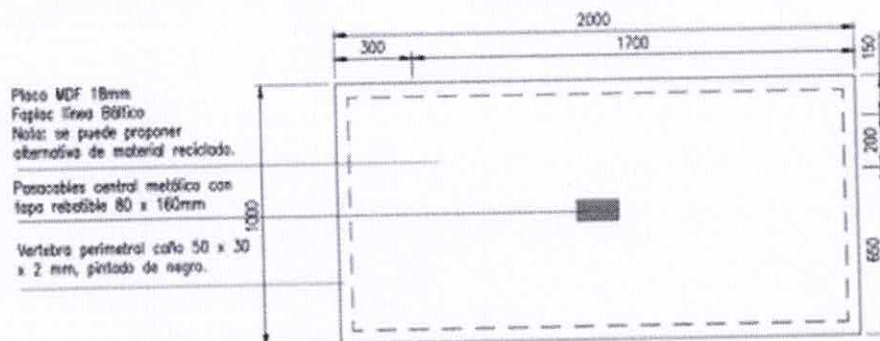
PLANTA MOBILIARIO D
