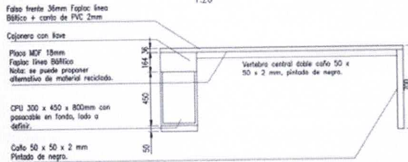
VISTA 1 MOBILIARIO A
