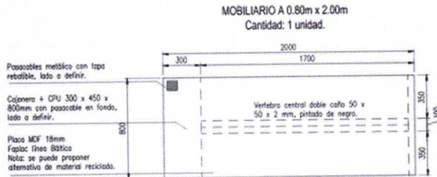
PLANTA MOBILIARIO A
