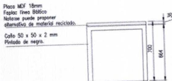
VISTA 2 MOBILIARIO C 1:20
