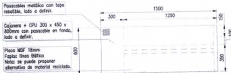
MOBILIARIO B 0.60m x 1.50m Cantidad: 15 unidades
