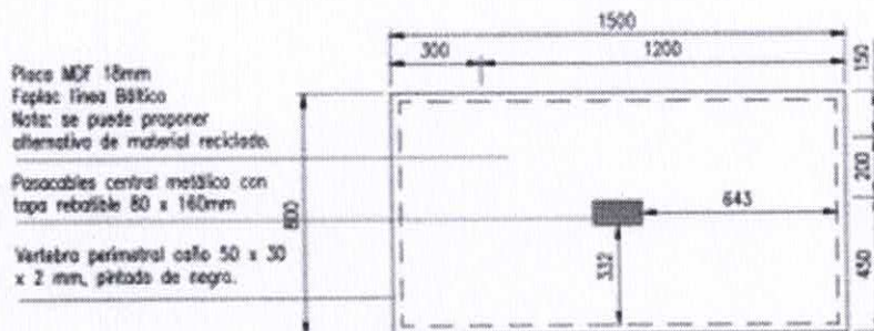
PLANTA MOBILIARIO E
