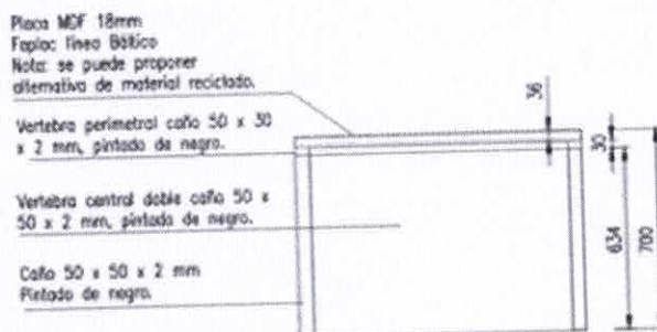
VISTA 2 MOBILIARIO D
