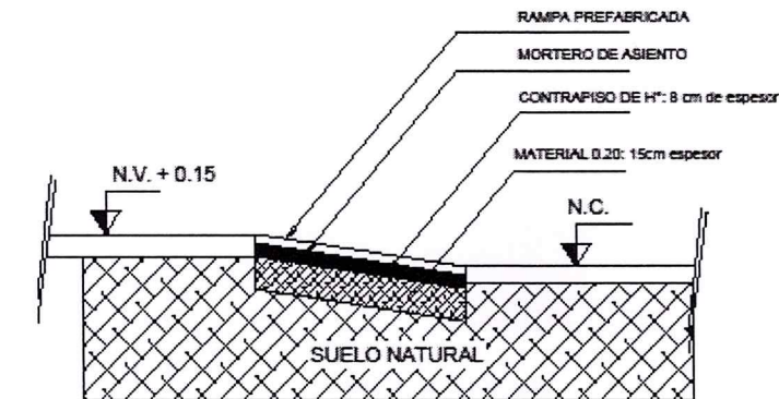
CORTE A-B
