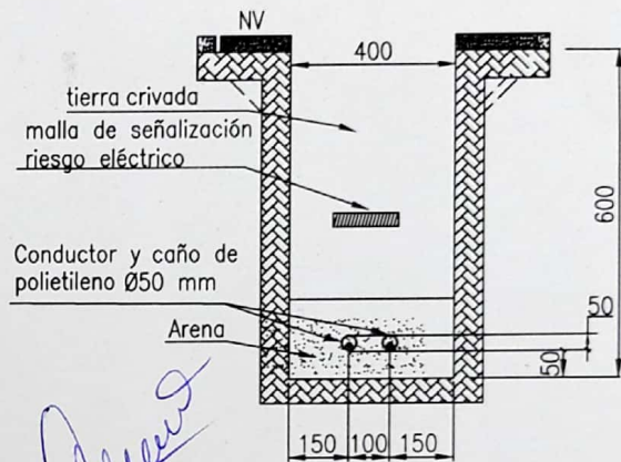
2 CONDUCTORES
