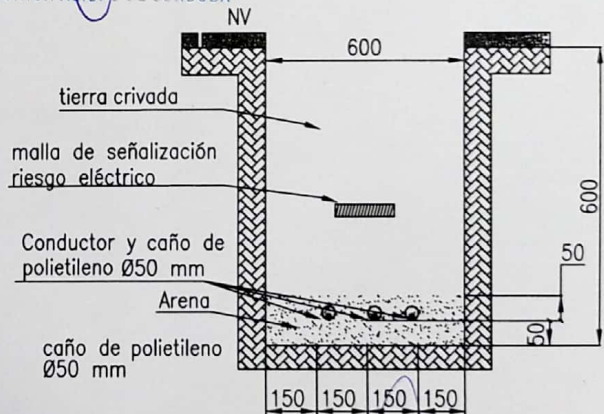
3 CONDUCTORES
