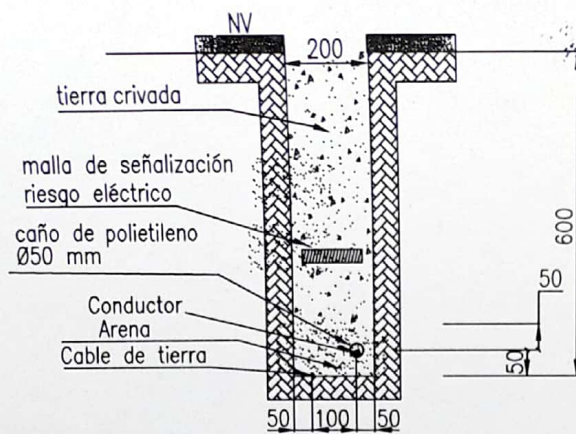
1 CONDUCTOR + CABLE DE TIERRA
