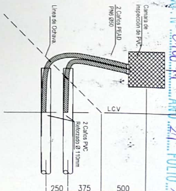
Detalle N°4
