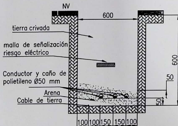
3 CONDUCTORES + CABLE DE TIERRA
