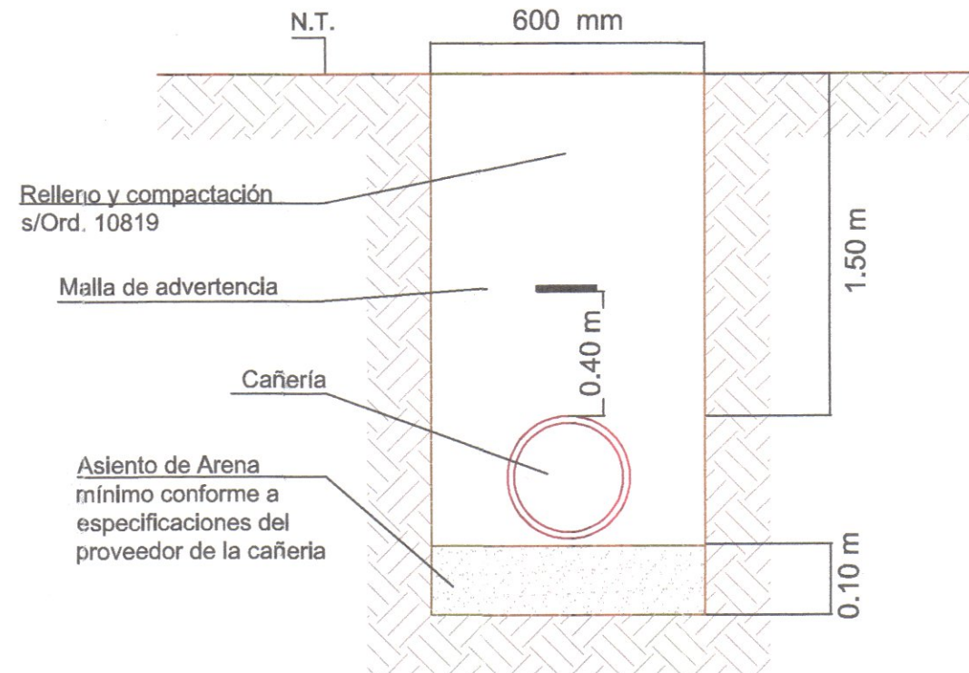
PERFIL DE ZANJA ZONA COLECTORA
