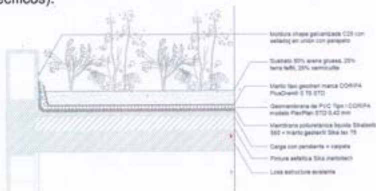
Ilustración 1 Detalle base cubierta ajardinada para canchales y gradas verdes
