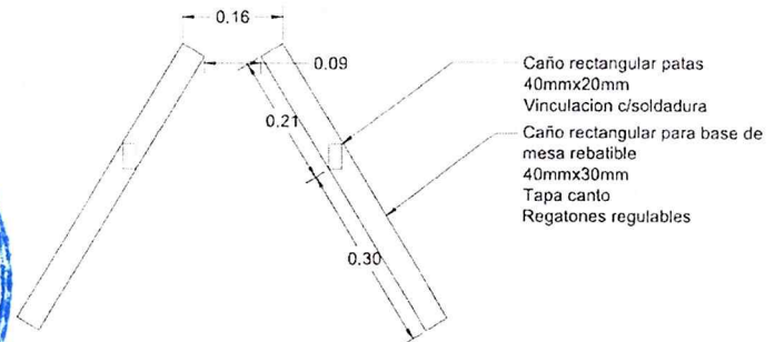
VISTA APOYO BASE
