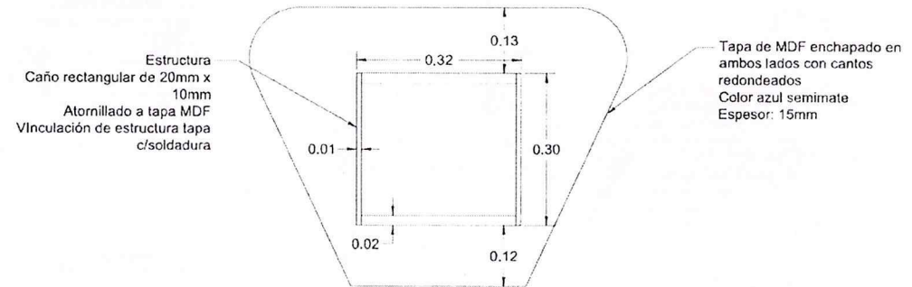
VISTA POSTERIOR TAPA
