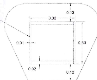
VISTA POSTERIOR TAPA
