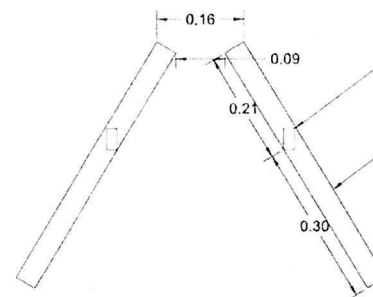
VISTA APOYO BASE
