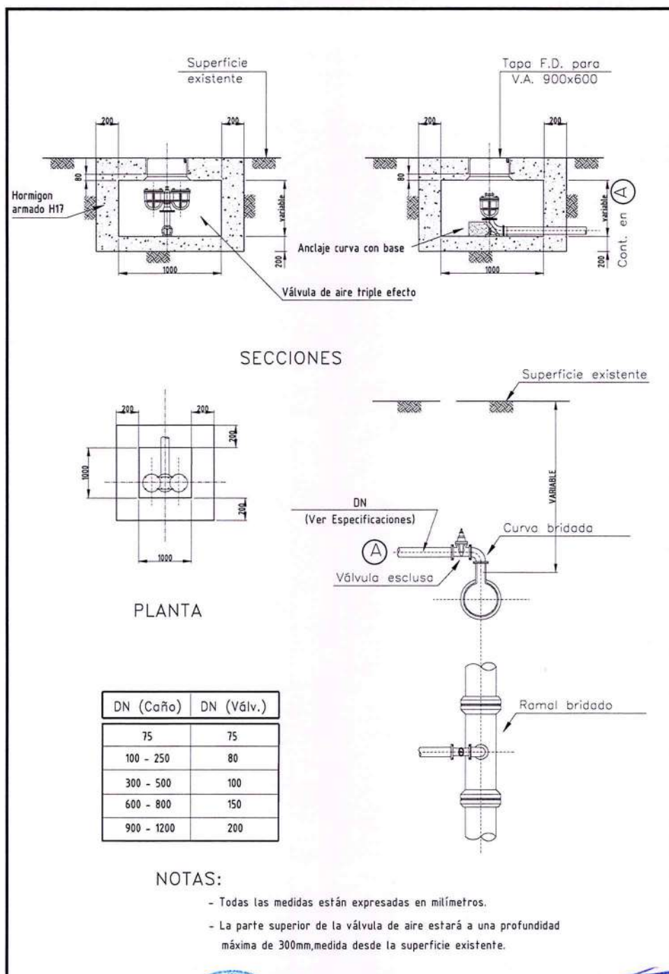
Figura 2: Plano tipo Válvula de aire
