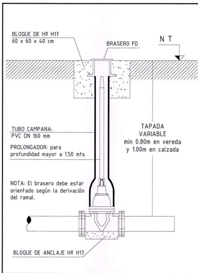
Figura 3: Plano tipo válvula esclusa
