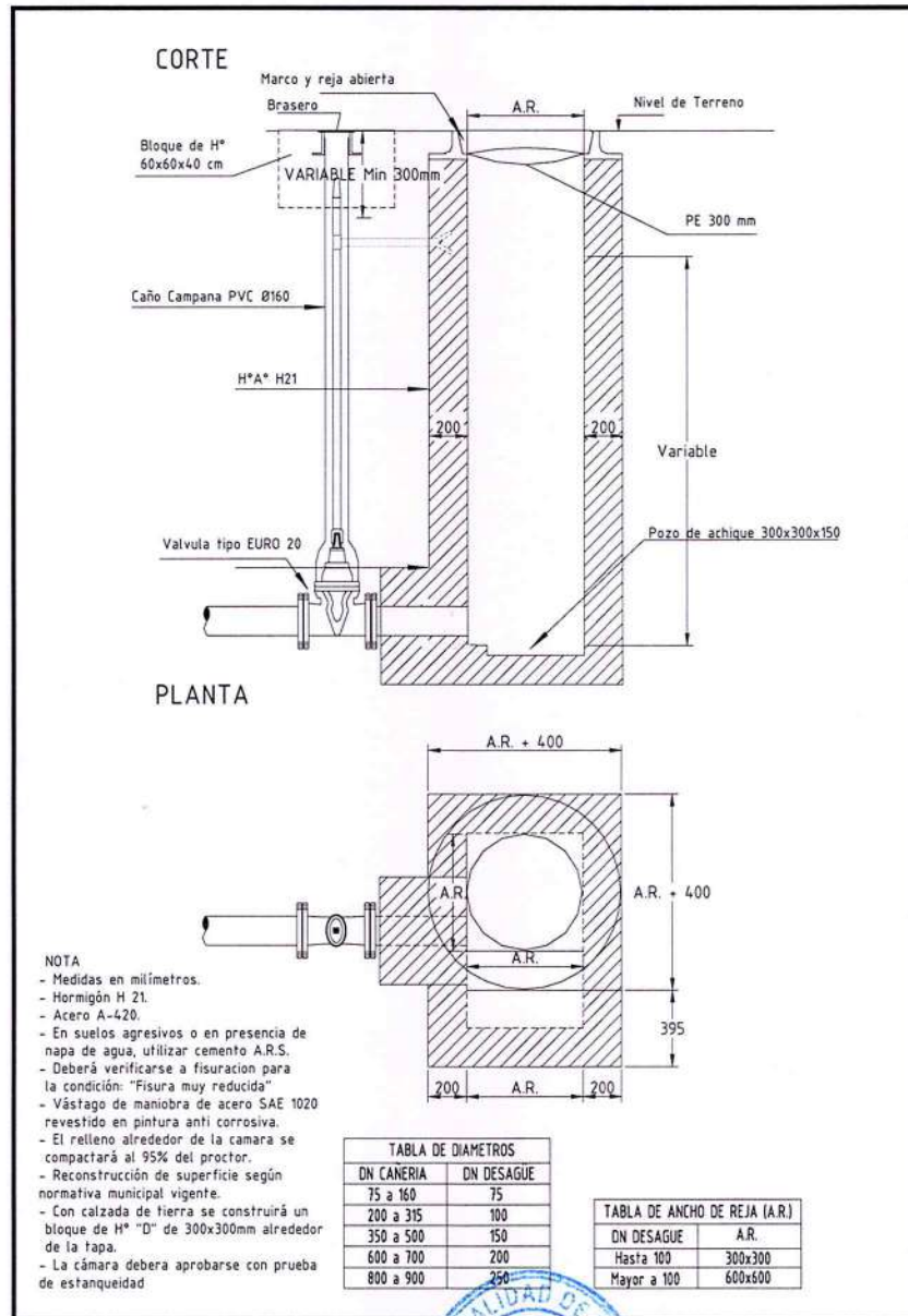
Figura 1: Plano tipo Cámara desagüe
