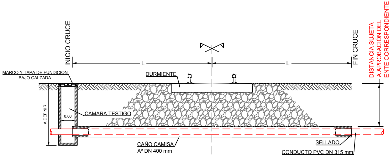
CORTE CRUCE FFCC
