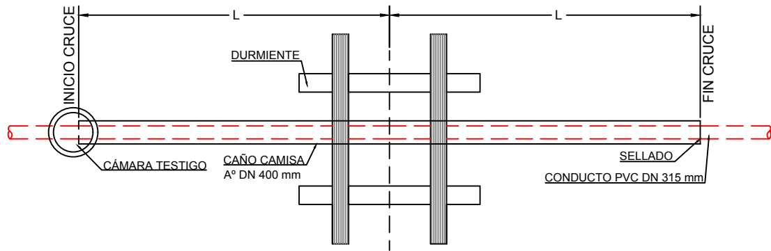
PLANTA CRUCE FFCC
