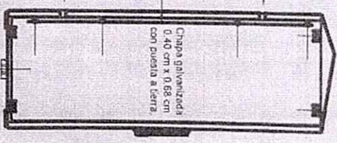
CORTE A-A
