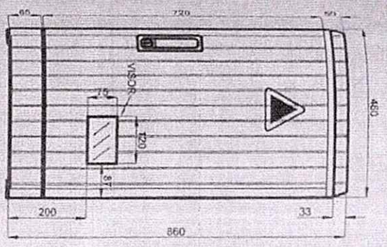
VISTA INFERIOR
