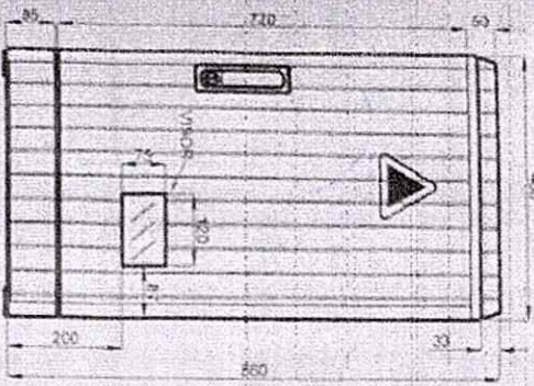
VISTA FRENTE
