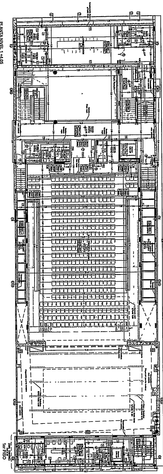
PLANTA NIVEL 1 +4.05
