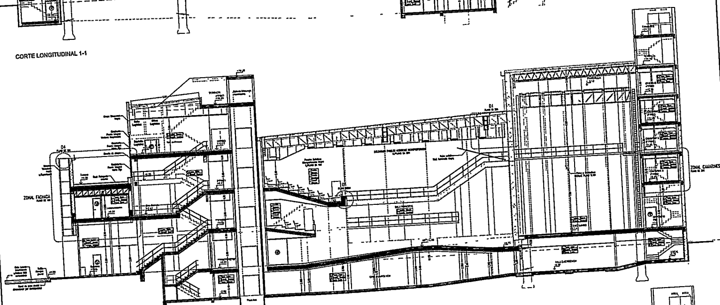
CORTE LONGITUDINAL 2-2
