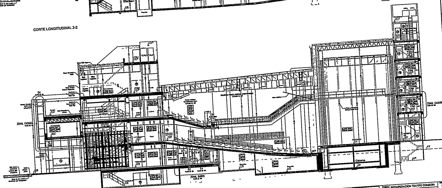
CORTE LONGITUDINAL 3-3
