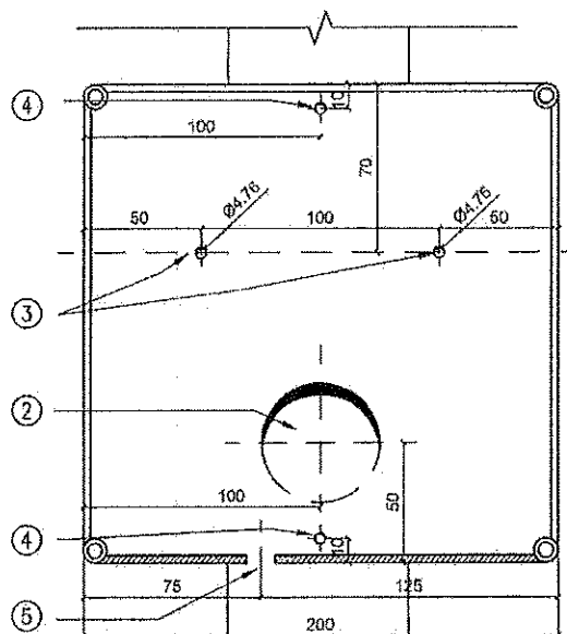
Corte transversal
