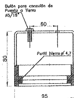
CORTE A-A
