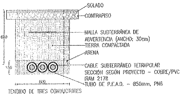
TENDIDO DE TRES CONDUCTORES
