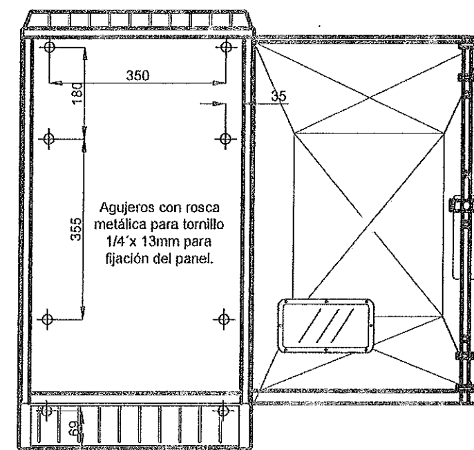
VISTA CON PUERTA ABIERTA
