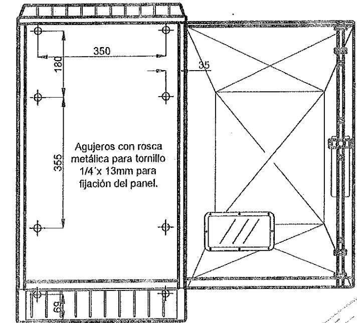
VISTA CON PUERTA ABIERTA
