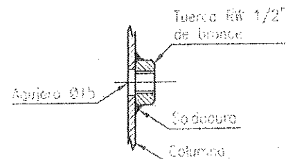
DETALLE "B" PUERTA A TIERRA
