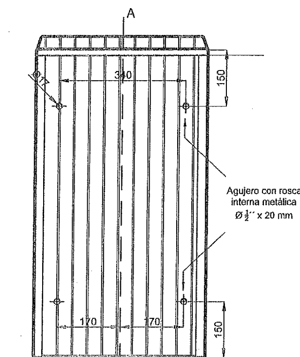
VISTA POSTERIOR (Ubicación de agujeros para instalar abrazadera)
