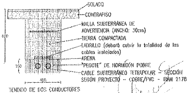
TENDIDO DE DOS CONDUCTORES
