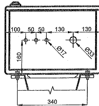
VISTA INFERIOR
