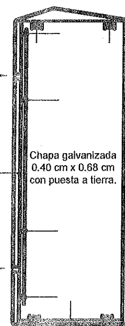
CORTE A-A
