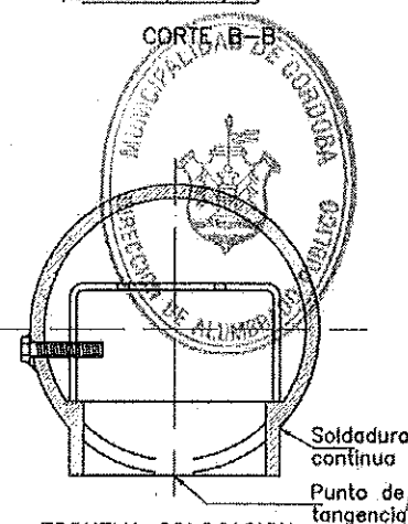
ESQUEMA COLOCACION DE CAJA EN COLUMNA
