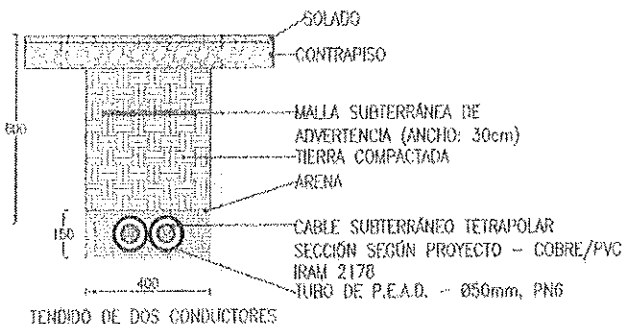
TENDIDO DE DOS CONDUCTORES
