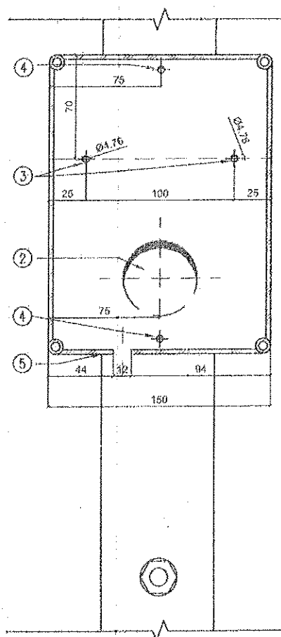
CORTE A-A
