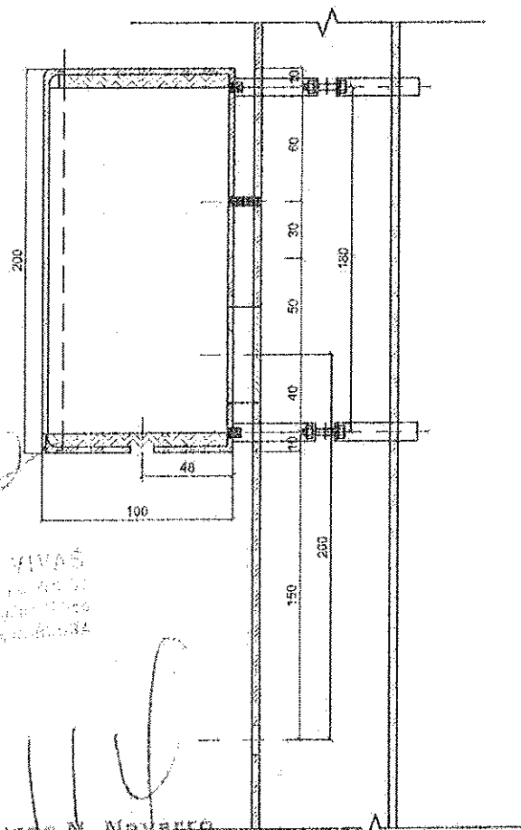
CORTE B-B
