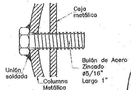
DETALLE "A" Bulón para conexión de Puesta a Tierra
