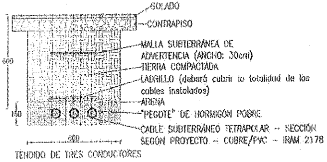
TENDIDO DE TRES CONDUCTORES
