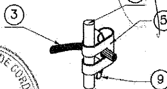
Detalle "B" (Conector tipo "TGC")
