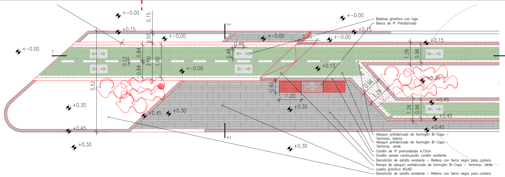
PLANTA 1:100
