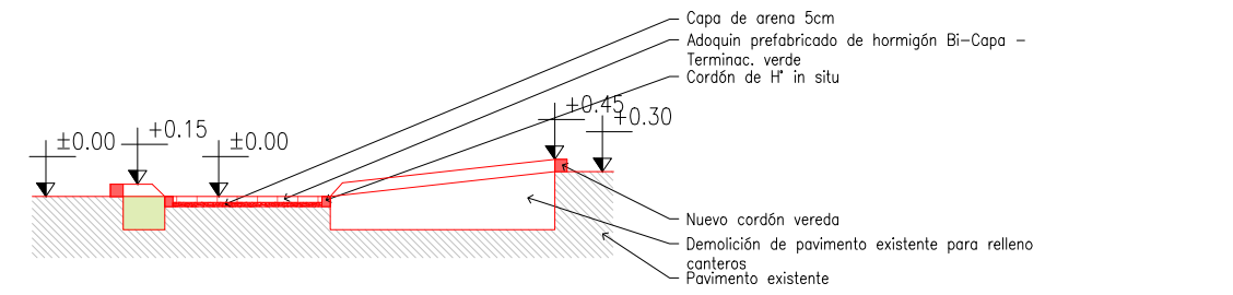
CORTE 2-2 1:100
