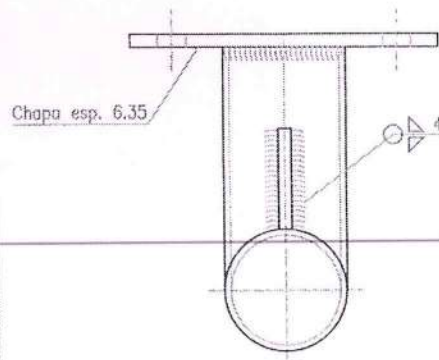
VISTA PLANTA
