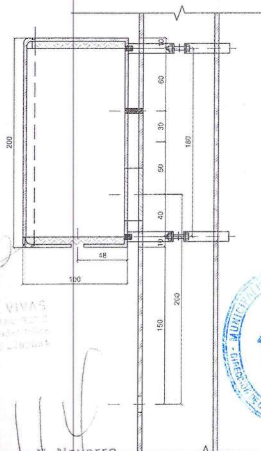
CORTE B-B
