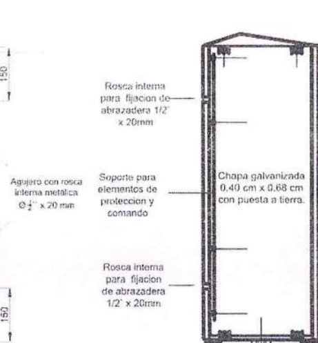
CORTE A-A
