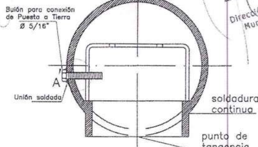
ESQUEMA COLOCACION DE CAJA EN COLUMNA
