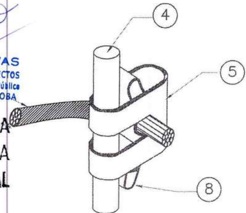
Detalle "B" (Conector tipo "TGC")
