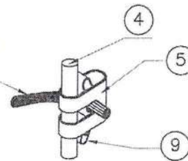
Detalle "B" (Conector tipo "TGC")
