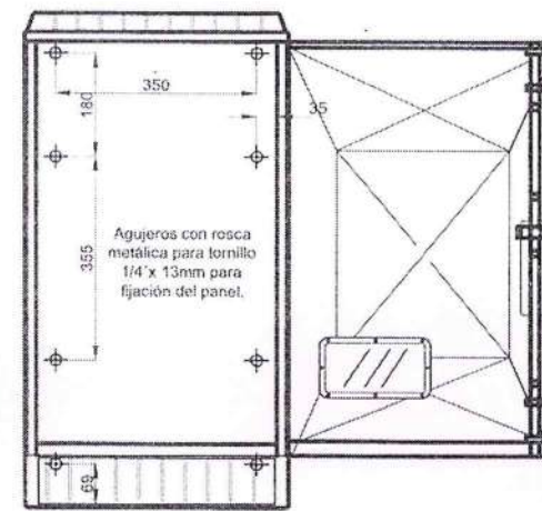
VISTA CON PUERTA ABIERTA
