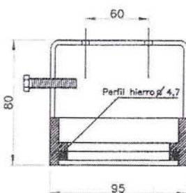
CORTE A-A
