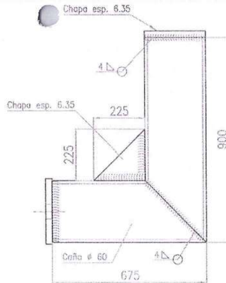
VISTA LATERAL
