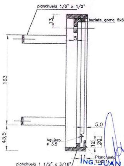
CORTE B-B
