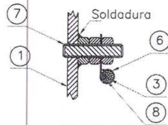
Detalle "A"
