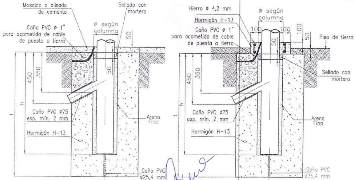
Corte A - A' Fundación para piso de mosaico o cemento alisado
