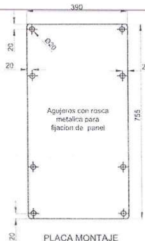
PLACA MONTAJE
