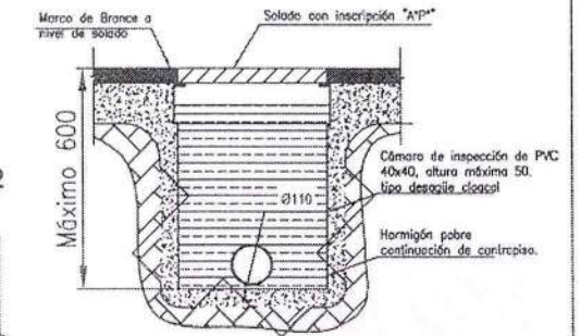
Cámara de paso para cruce de calle
