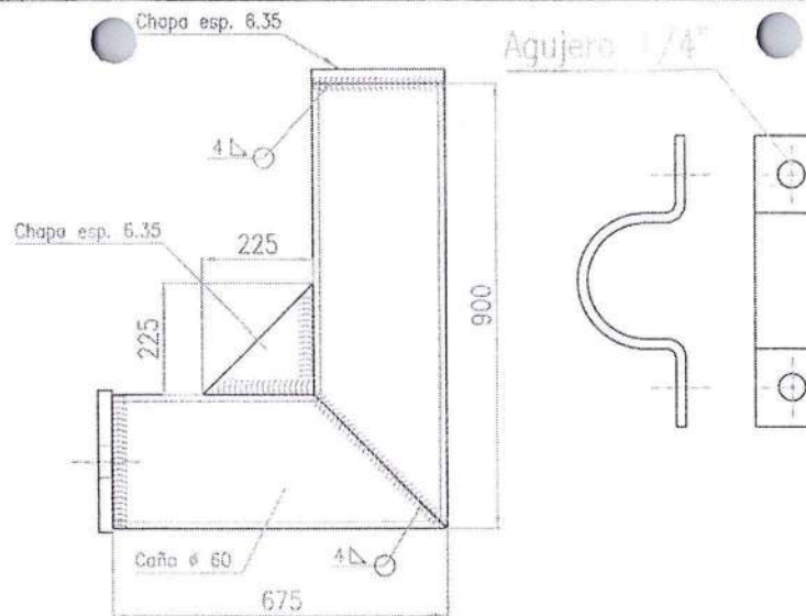
VISTA LATERAL
