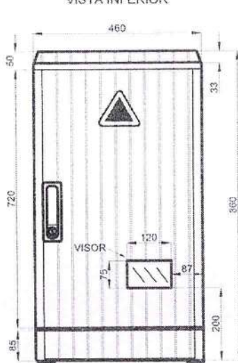
VISTA FRENTE
