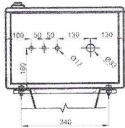
VISTA INFERIOR
