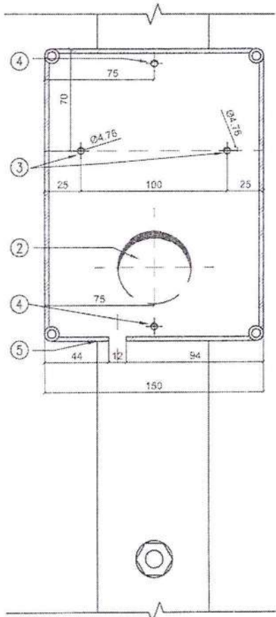
CORTE A-A
